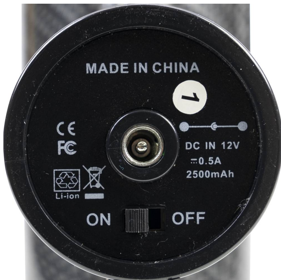
Bază aparat - date tehnice și alimentare
