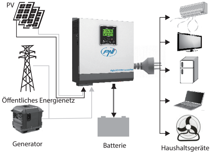
Bild. 1 Hybrid-Antriebssystem
