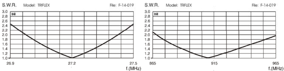
Raspuns SWR tipic
